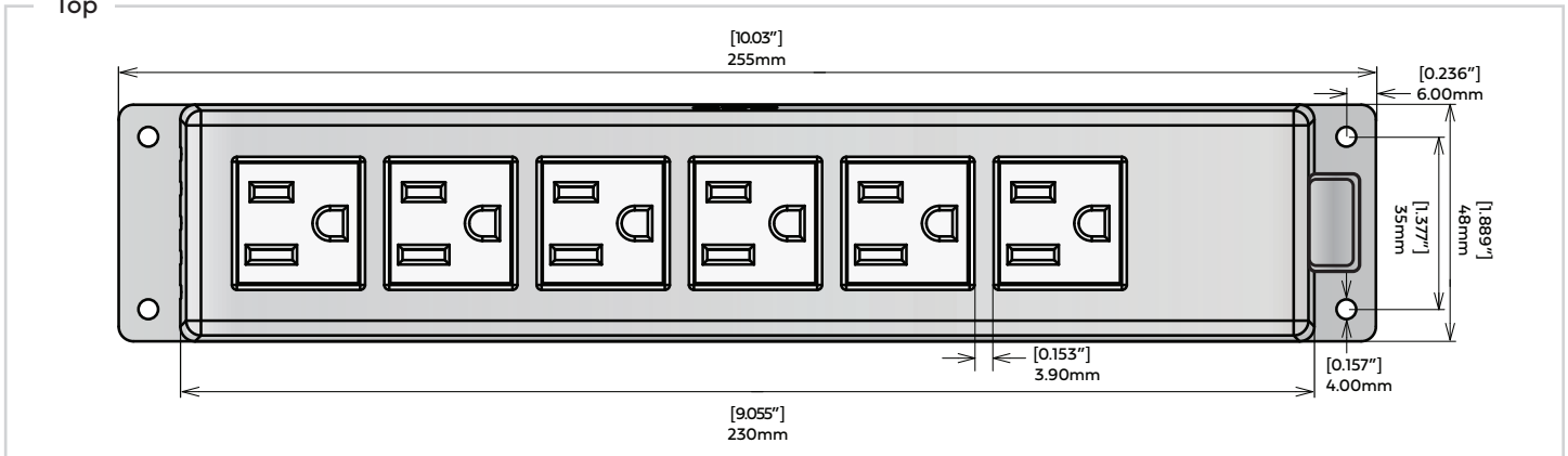
Top
